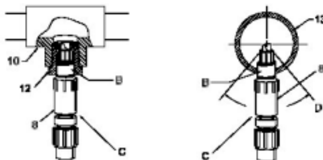
Obr. 2.2b Vstříkovací zpětný ventil
